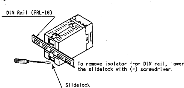
Fig.3 DIN Rail Mounting
